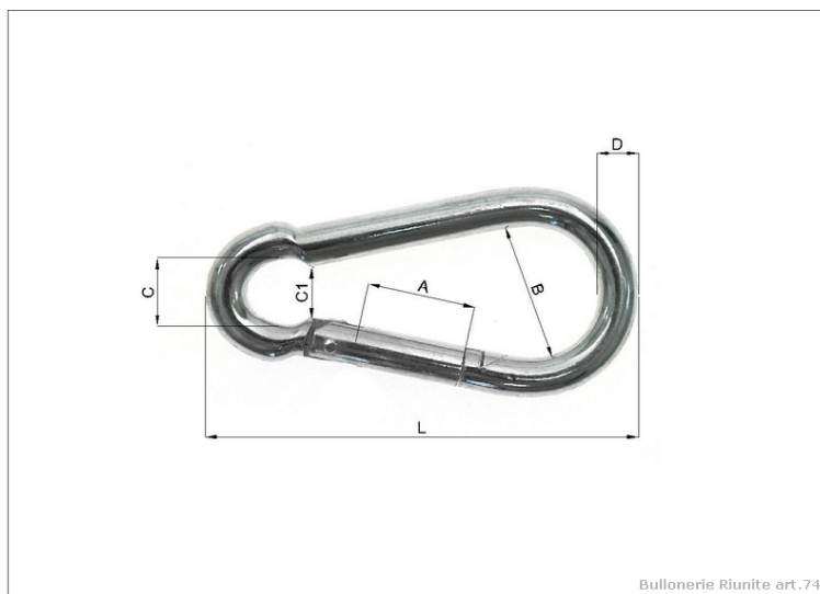
Bullonerie Riunite art.74
